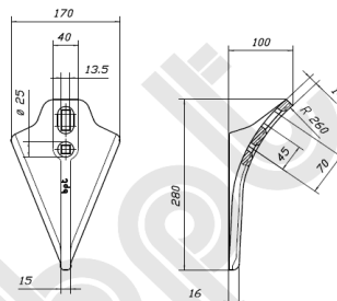
COD. 11139 VOMERE TIPO BELGIO SCHAR "BELGIO" POINT TYPE "BELGIO"
