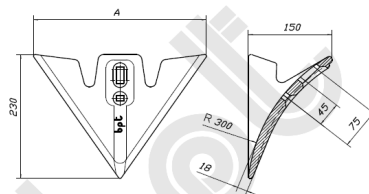
COD. A 11170 310 11420 420 VOMERE ZAMPA D'OCA GANSEFUSSSCHAR DUCK FOOT POINT
