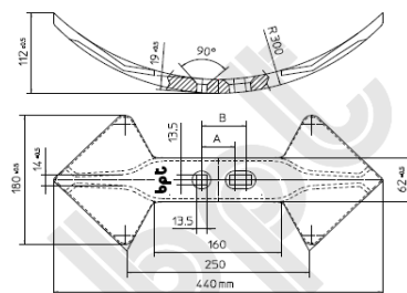
DOPPIO CUORE 180 mm - DOUBLE HEART POINT 180 mm - DOPPELHERZSCHAR 180 mm
